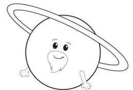
Uranus
