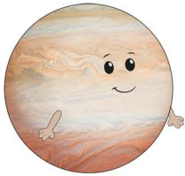
Jupiter
