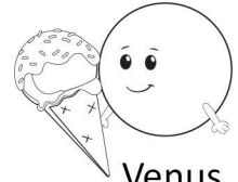
Venus
